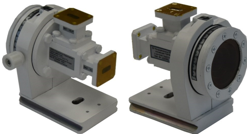
Рисунок 1 – Внешний вид облучателя
